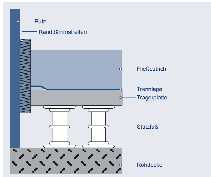
Abb. 13: Aufbau des Hohlraumbodens
