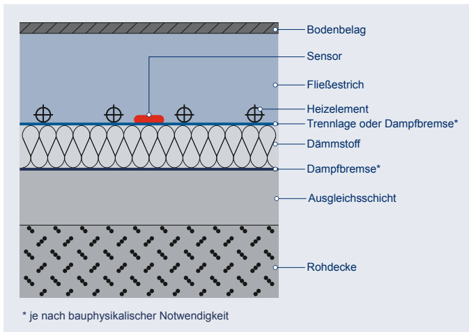
Abb. 16: Positionierung
