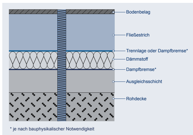
Abb. 2: Bewegungsfuge
