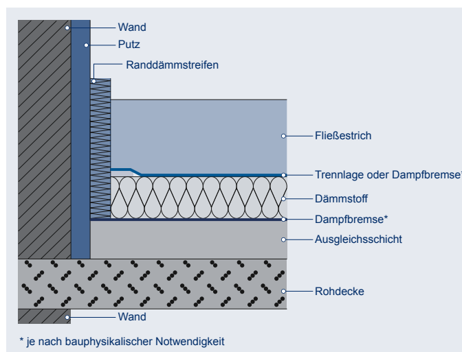
Abb. 9: schwimmender Estrich
