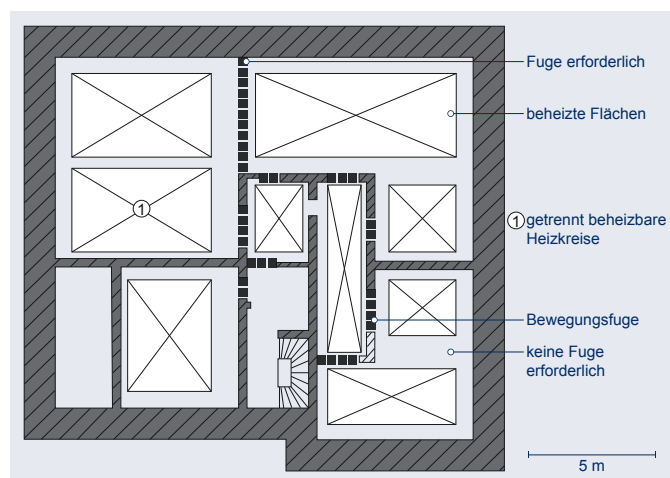
Abb. 4: Flächenaufteilung durch Feldfugen
