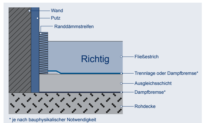
Abb. 5.4: saubere Randausbildung
