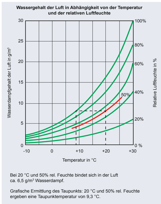
Abb. 15: Wassergehalt
